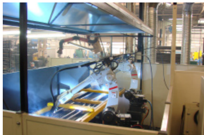
Fot. 14. Stanowisko do spawania pomostów
