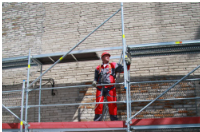
Fot. 12. Montaż zestawu bezpieczeństwa
