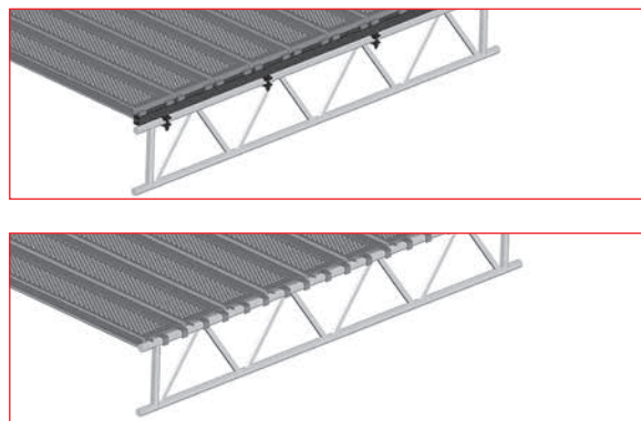
Рис. 3.37 – Монтаж траверса на ферме
