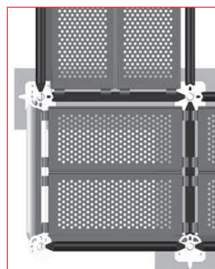
Рис. 3.25 - Угол, выполненный при помощи трех стоек, опоры и связи (см. рис. 3.28)
