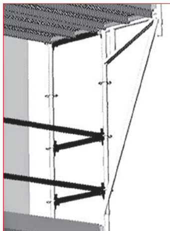
Рис. 3.28 – Расширение с помощью опоры 0,73 м и связи
