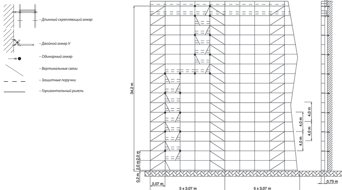
Схема анкеровки проходной вертикали
